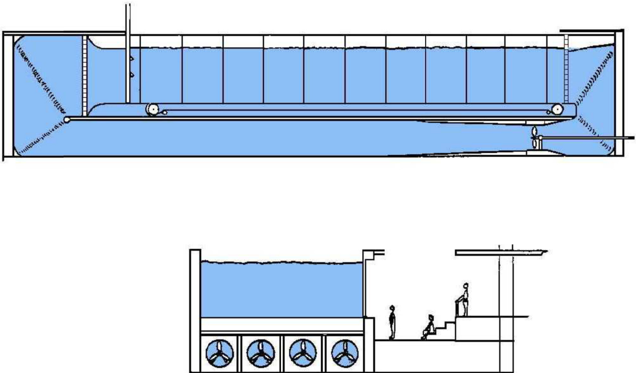
Figur 8: Skisse av SINTEFs strømningstank i Hirtshals. Øverst: sett fra siden, nederst: sett forfra. (SINTEF, 2011)
